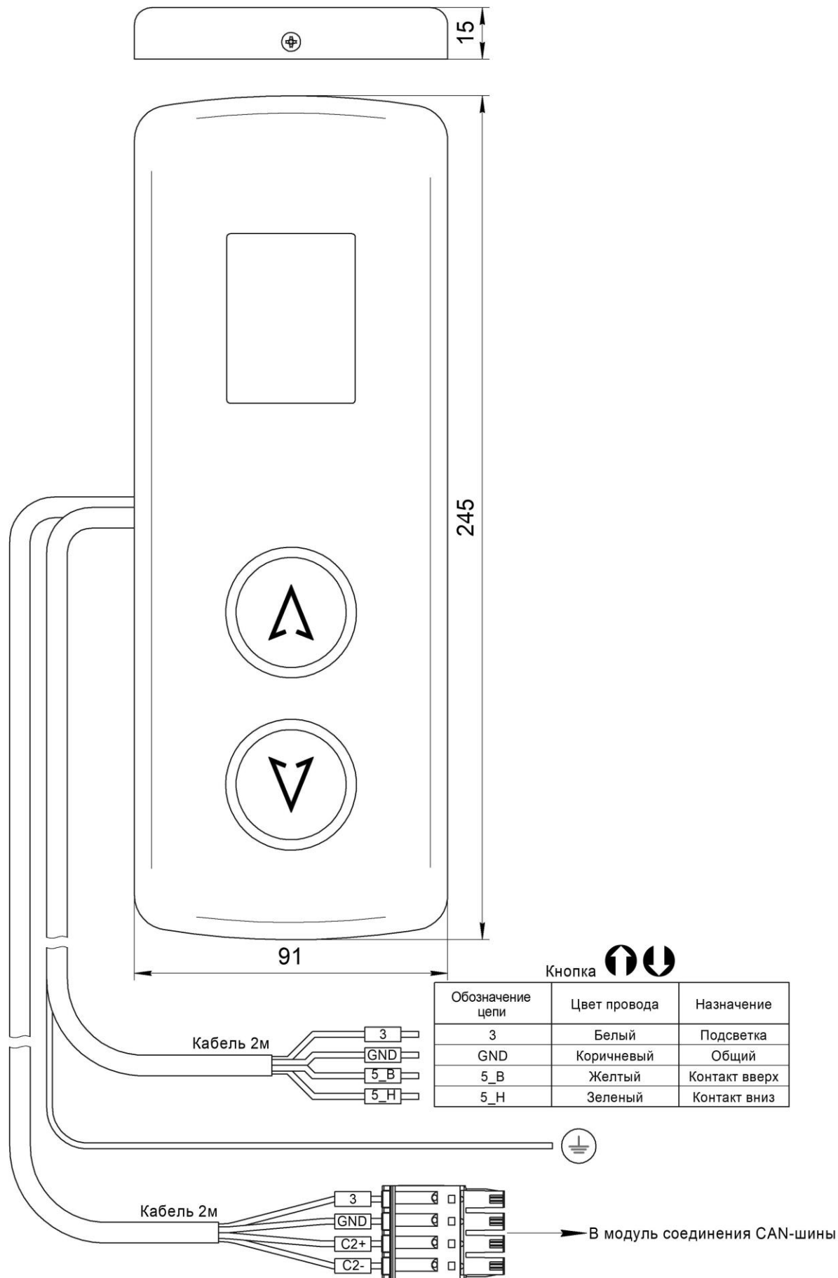
Рис.1 Внешний вид, габаритные и установочные размеры Вызывного поста ЦИРКОН НШЕК.468381.021
